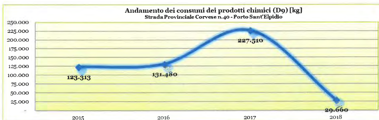
FIGURA 25: ANDAMENTO CONSUMO PRODOTTI CHIMICI IMPIANTO DI TRATTAMENTO CHIMICO FISICO (D9)
